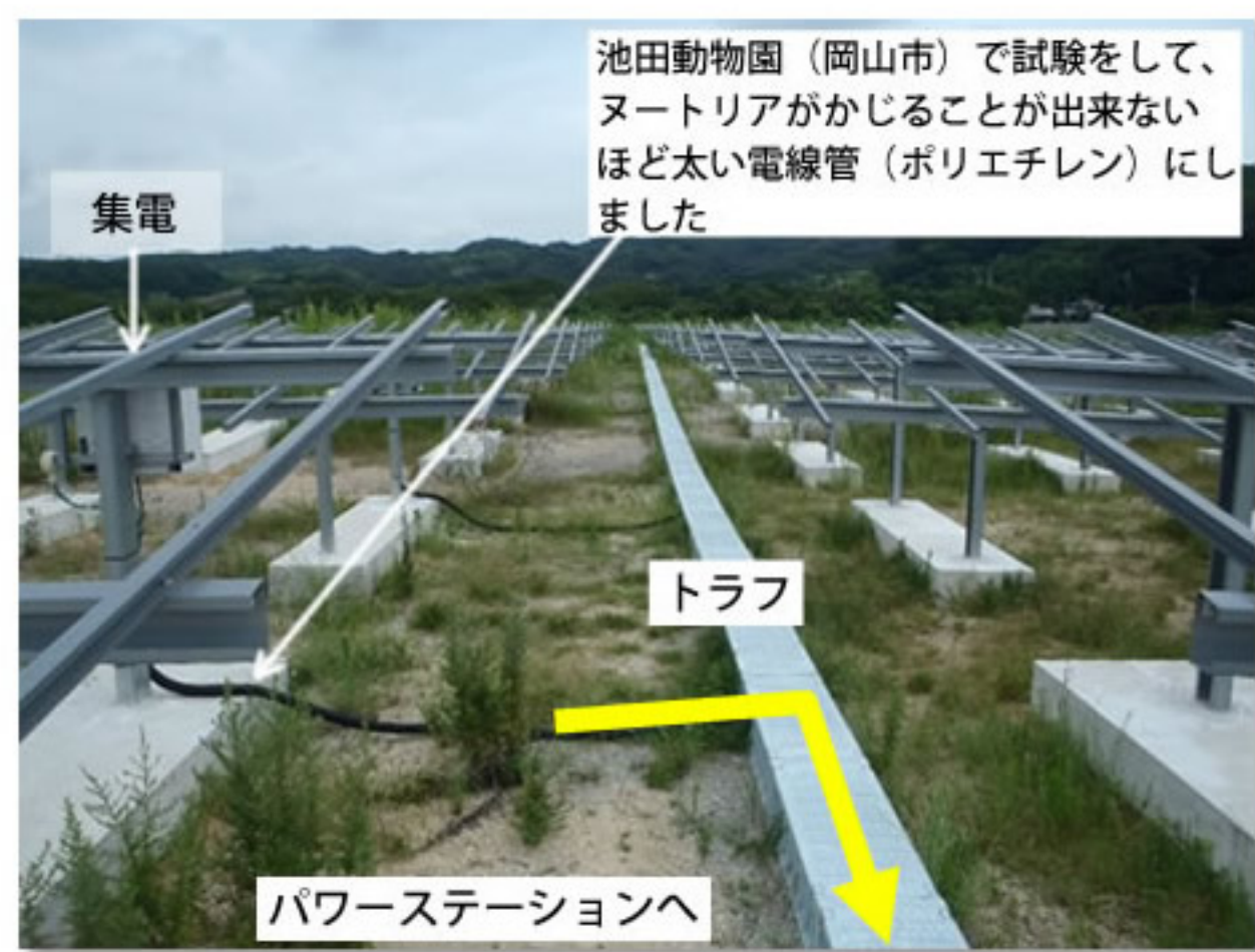
③ 集電箱からトラフへ
